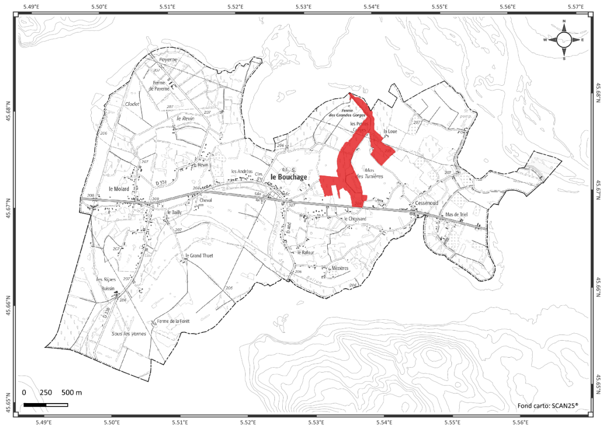
▲ En rouge : zone humide des Petites Gorges, hotspot de biodiversité
